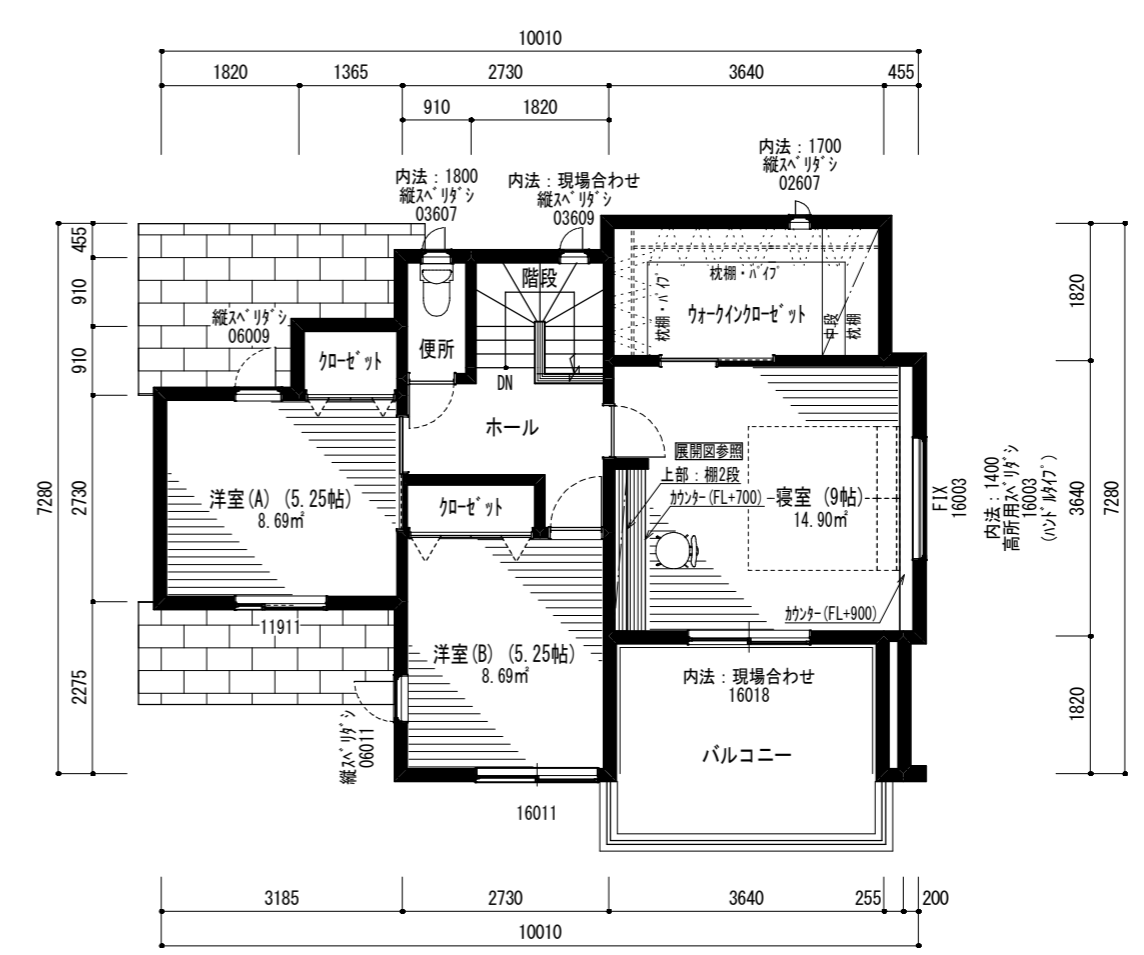
2階平面図 (プレゼン) 1/100
