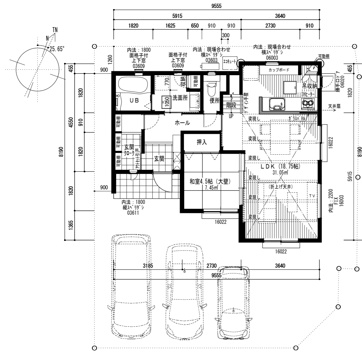
1階平面図 (プレゼン) 1/100
