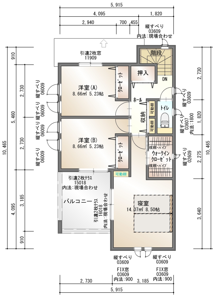
2階平面図
