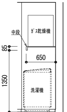
ガス乾燥機スレス断面図 1/50
