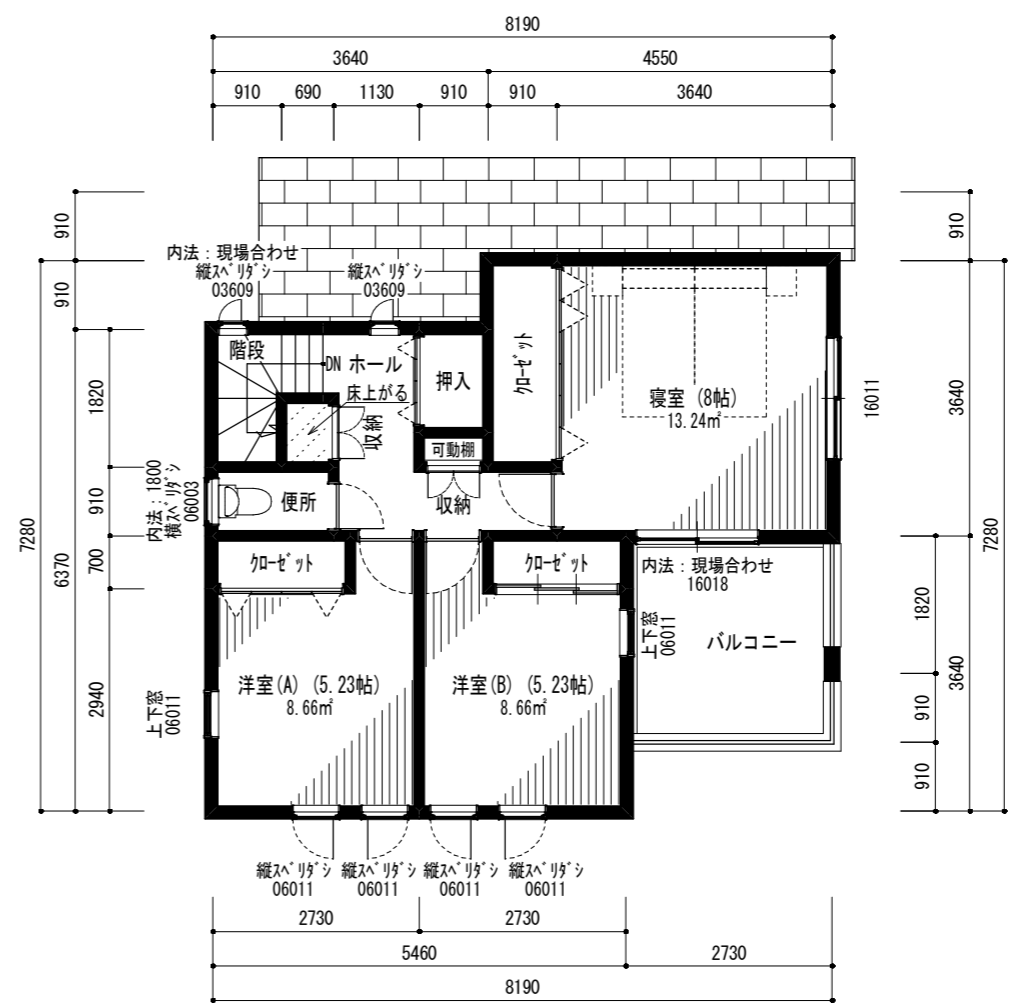
2階平面図 (プレゼン) 1/100
