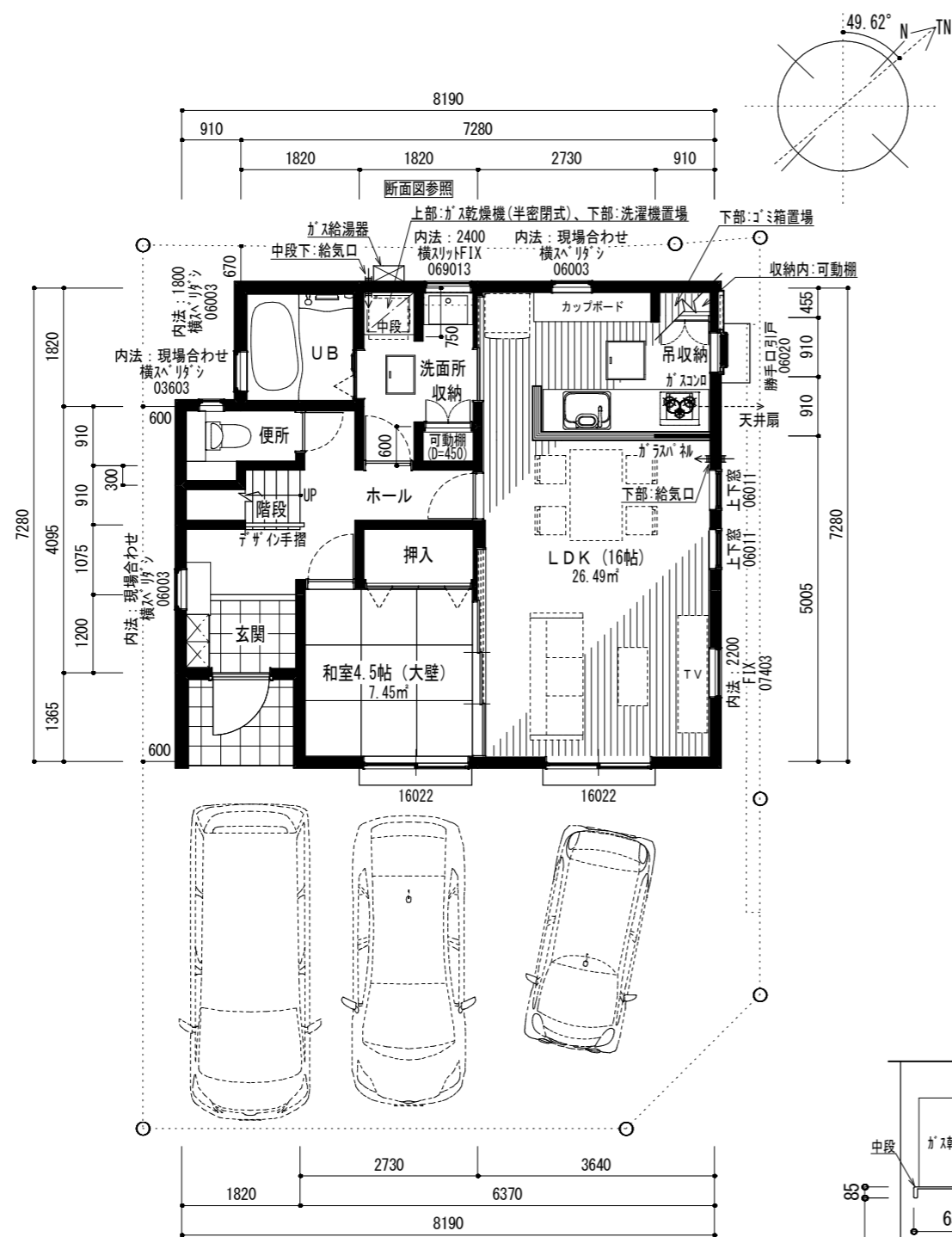
1階平面図 (プレゼン) 1/100
