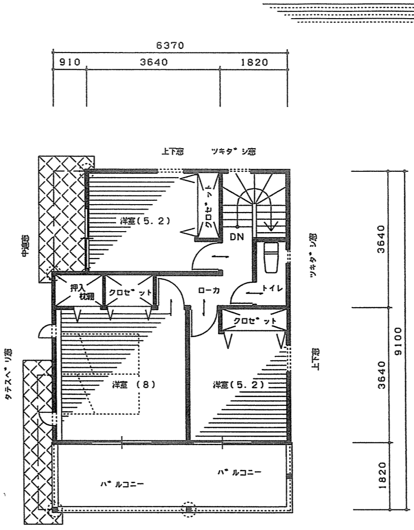
2階 平面図 1/100
