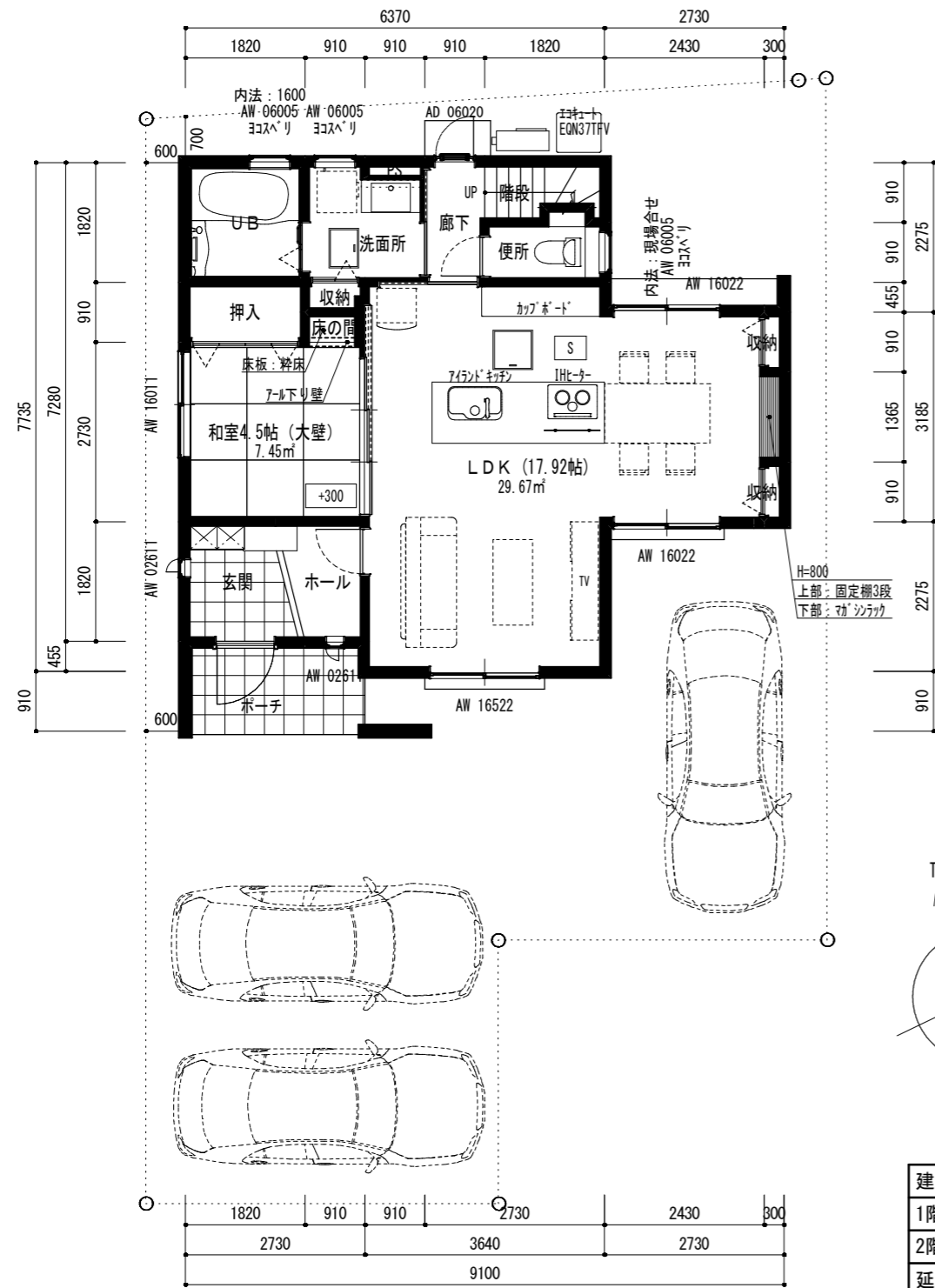
1階平面図 (プレゼン) 1/100
