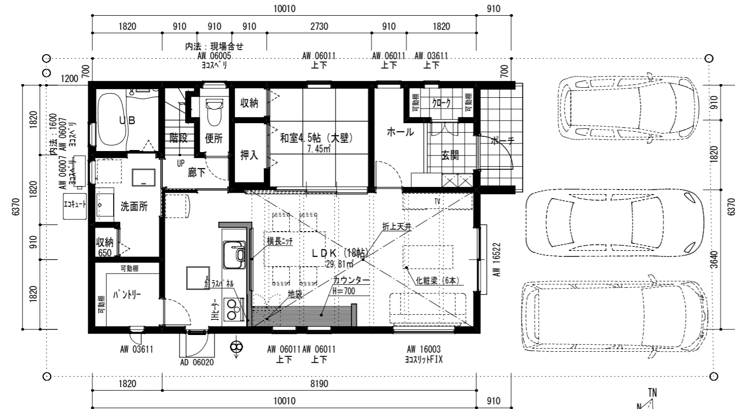
1階平面図 (プレゼン) 1/100
