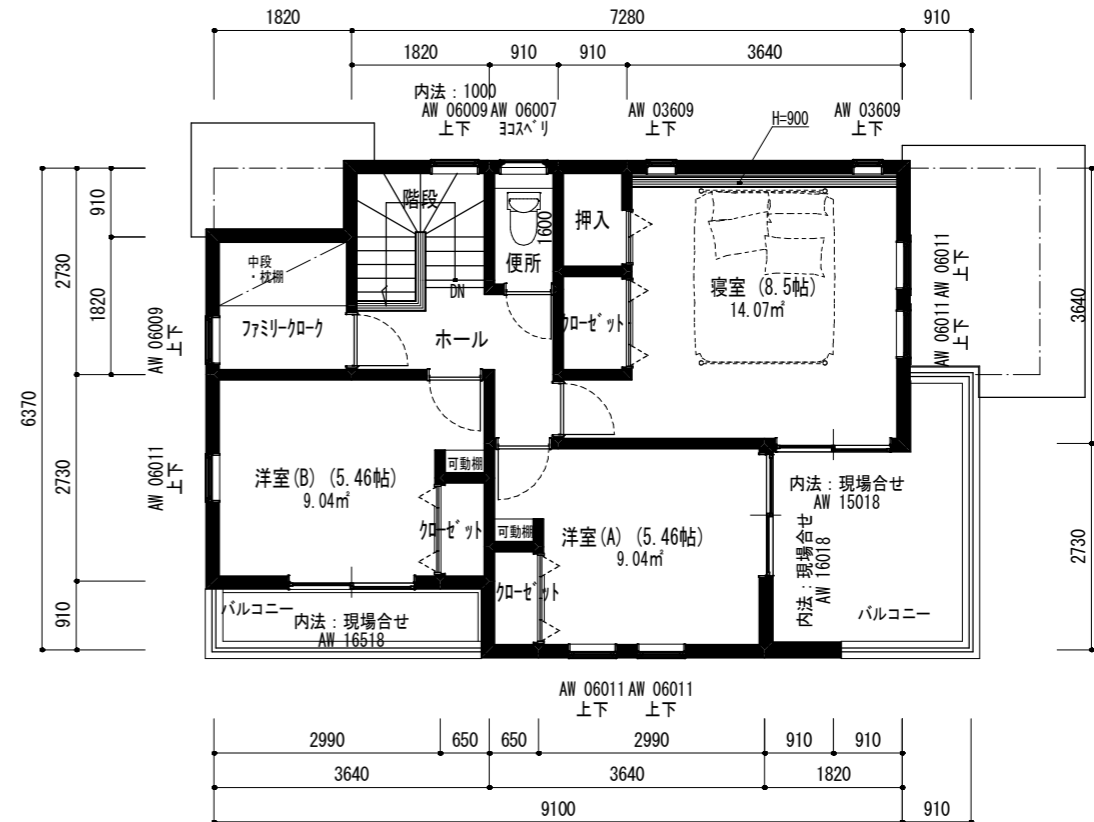
2階平面図 (プレゼン) 1/100
