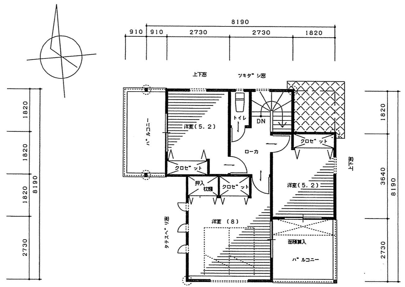
2階 平面図
