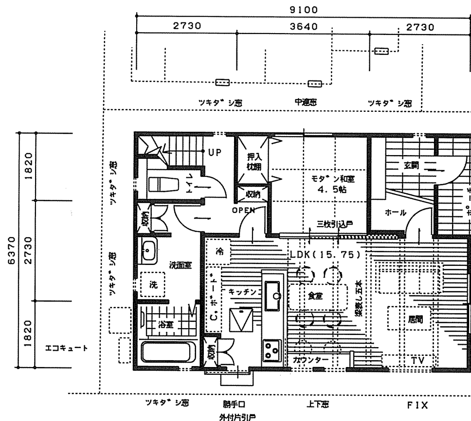
1階 平面図
