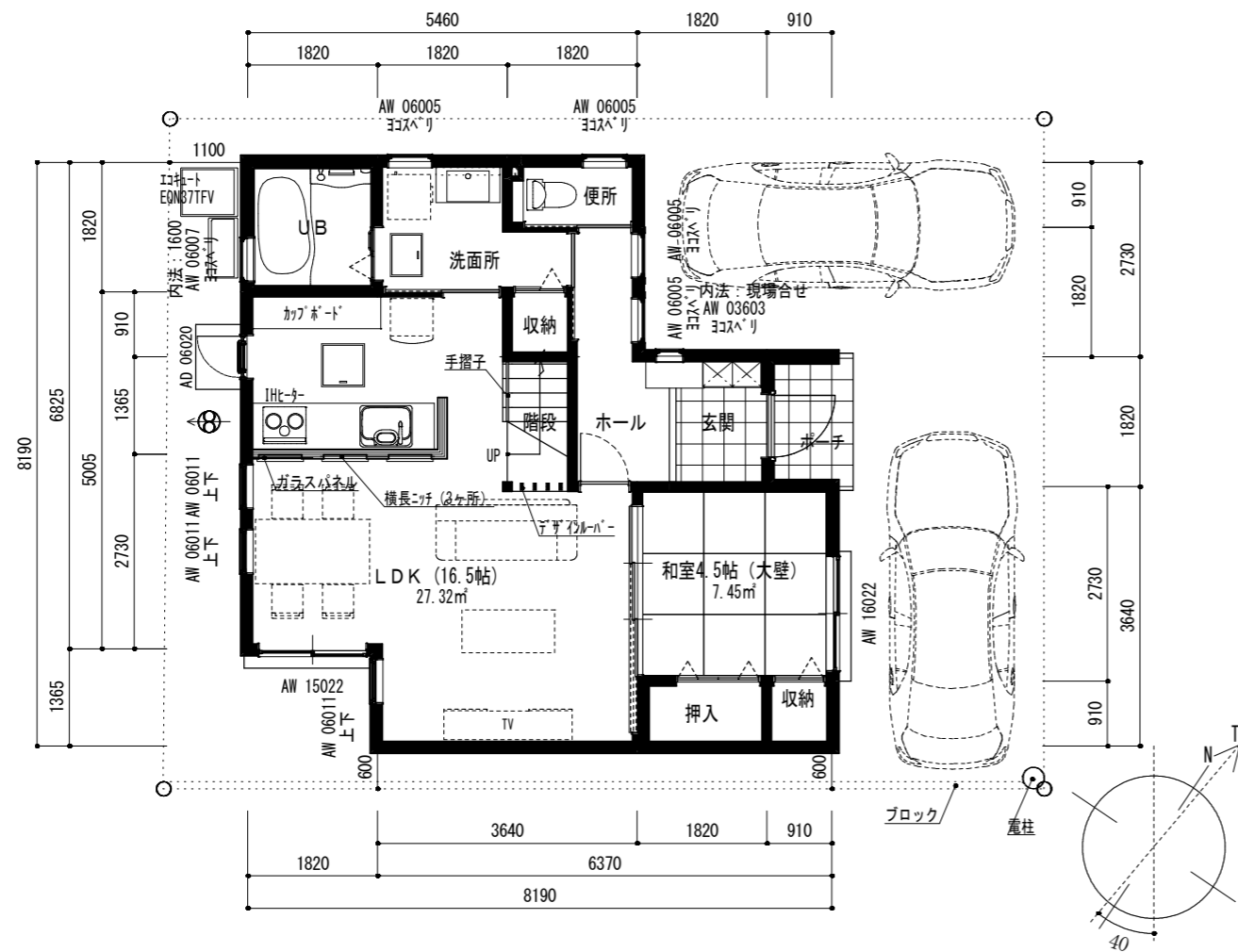
1階平面図 (プレゼン) 1/100
