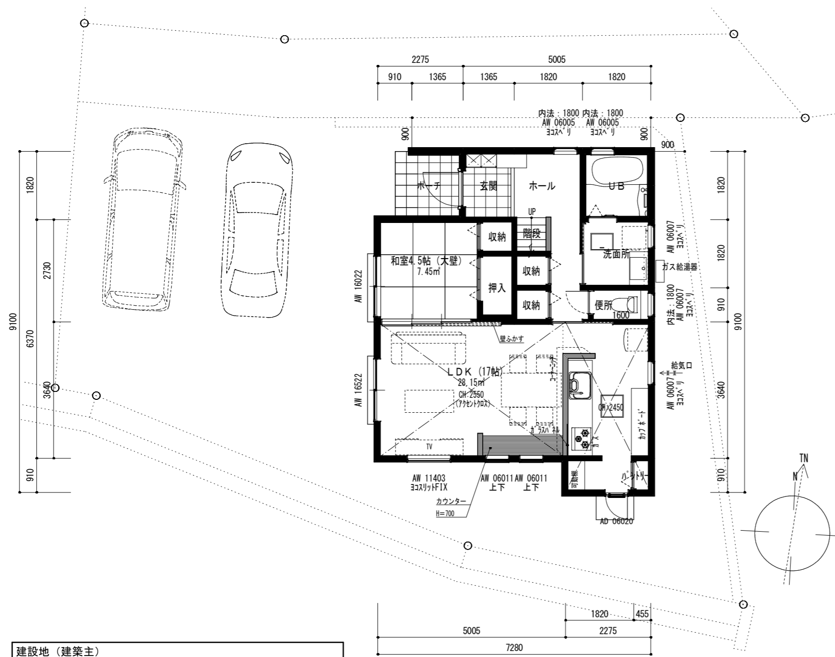
1階平面図 (プレゼン用) 1/100
