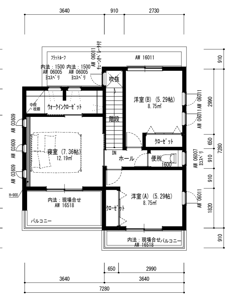
2階平面図 (プレゼン用) 1/100
