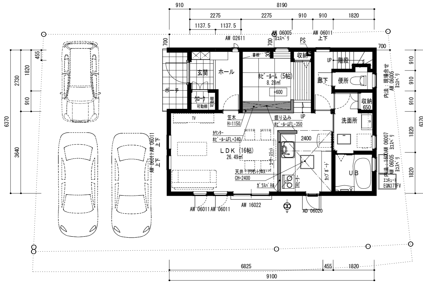
1階平面図 (プレゼン用) 1/100
