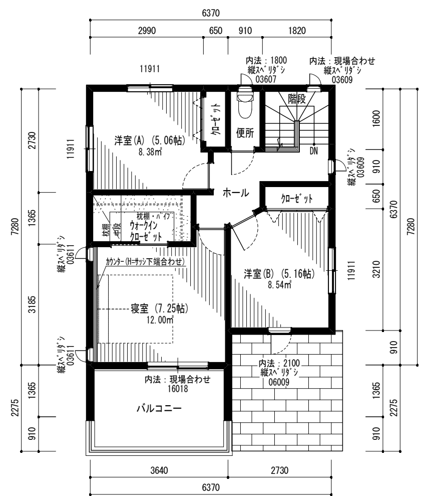
2階平面図 (プレゼン) 1/100
