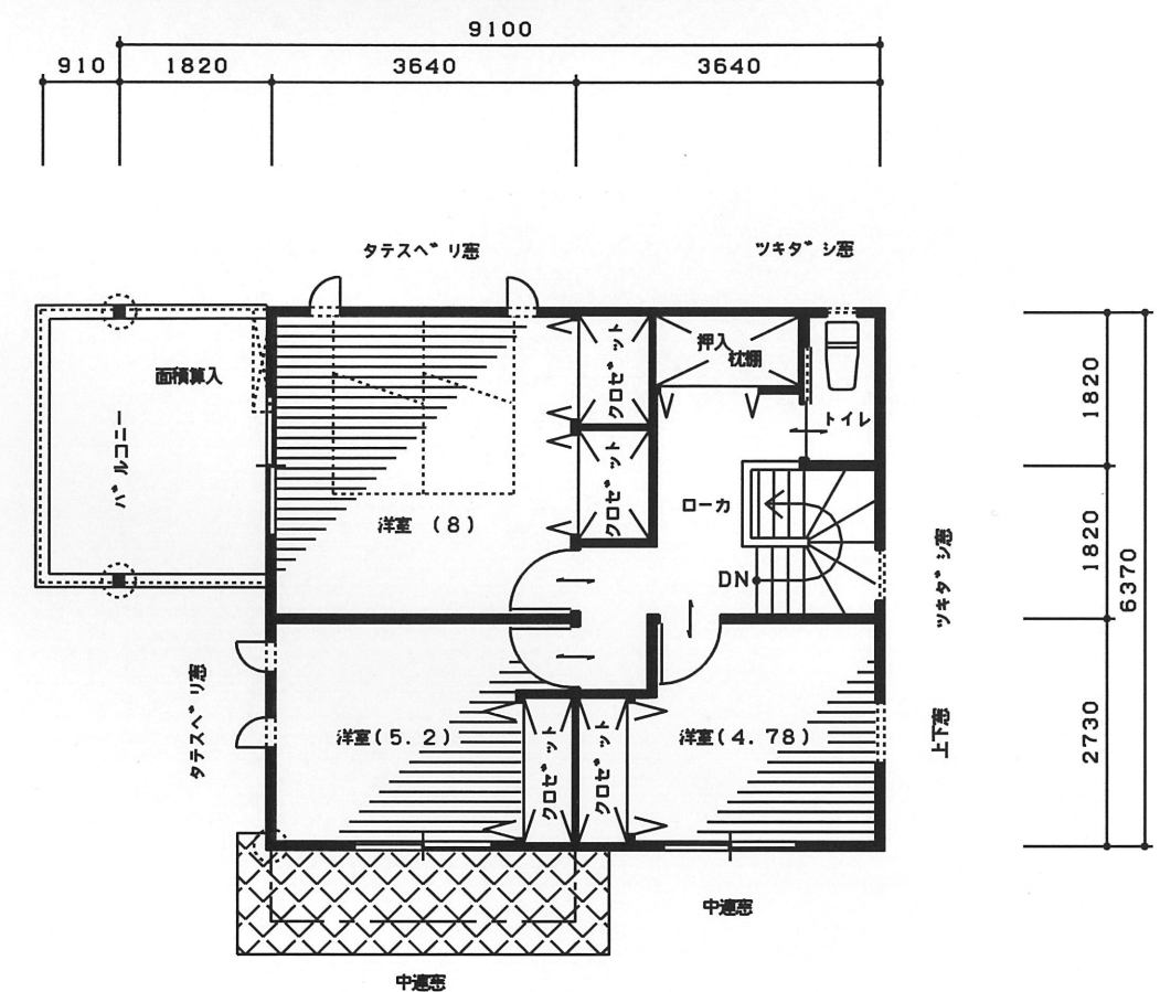
2階 平面図 1/100
