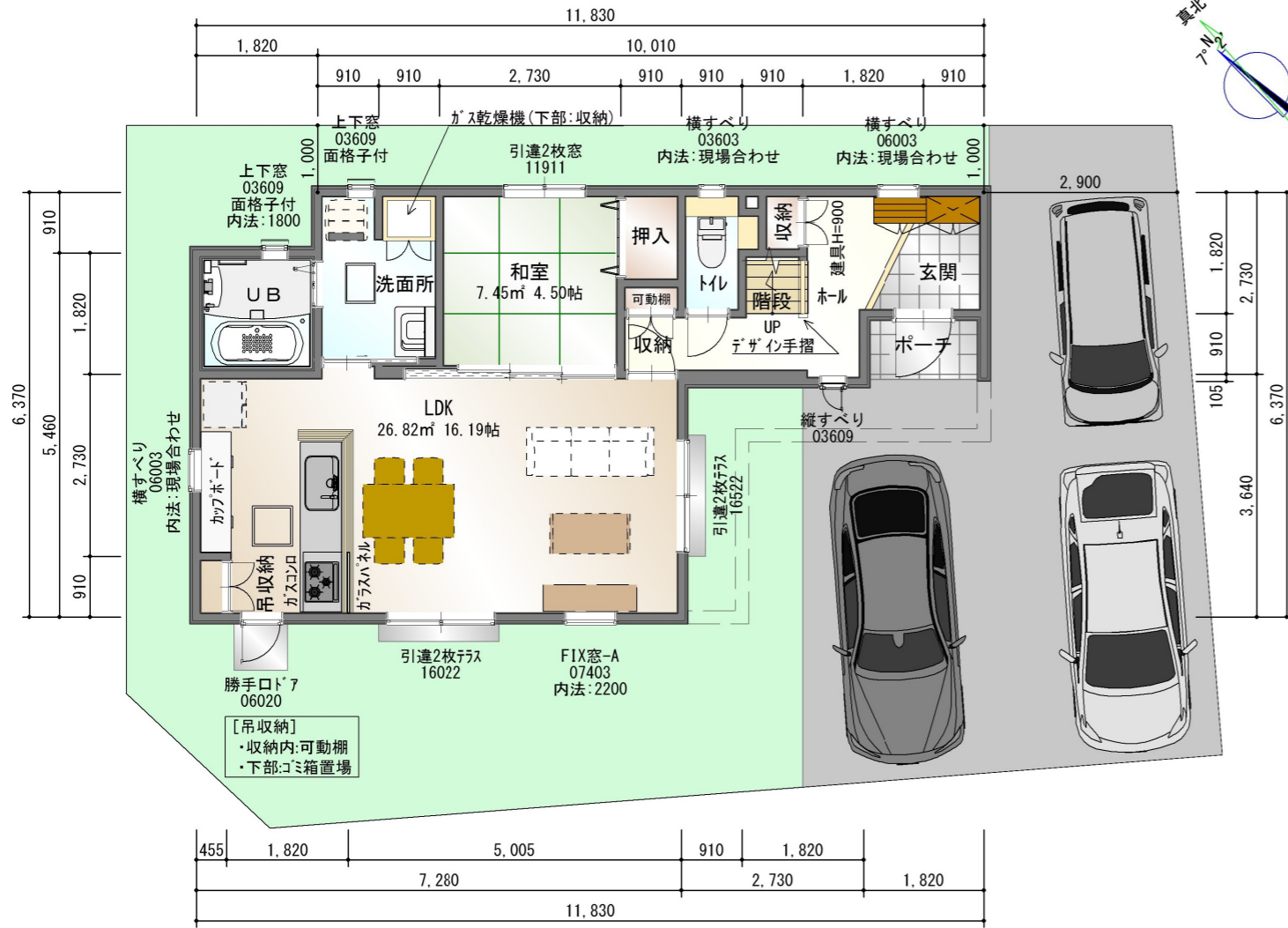
1階平面図
