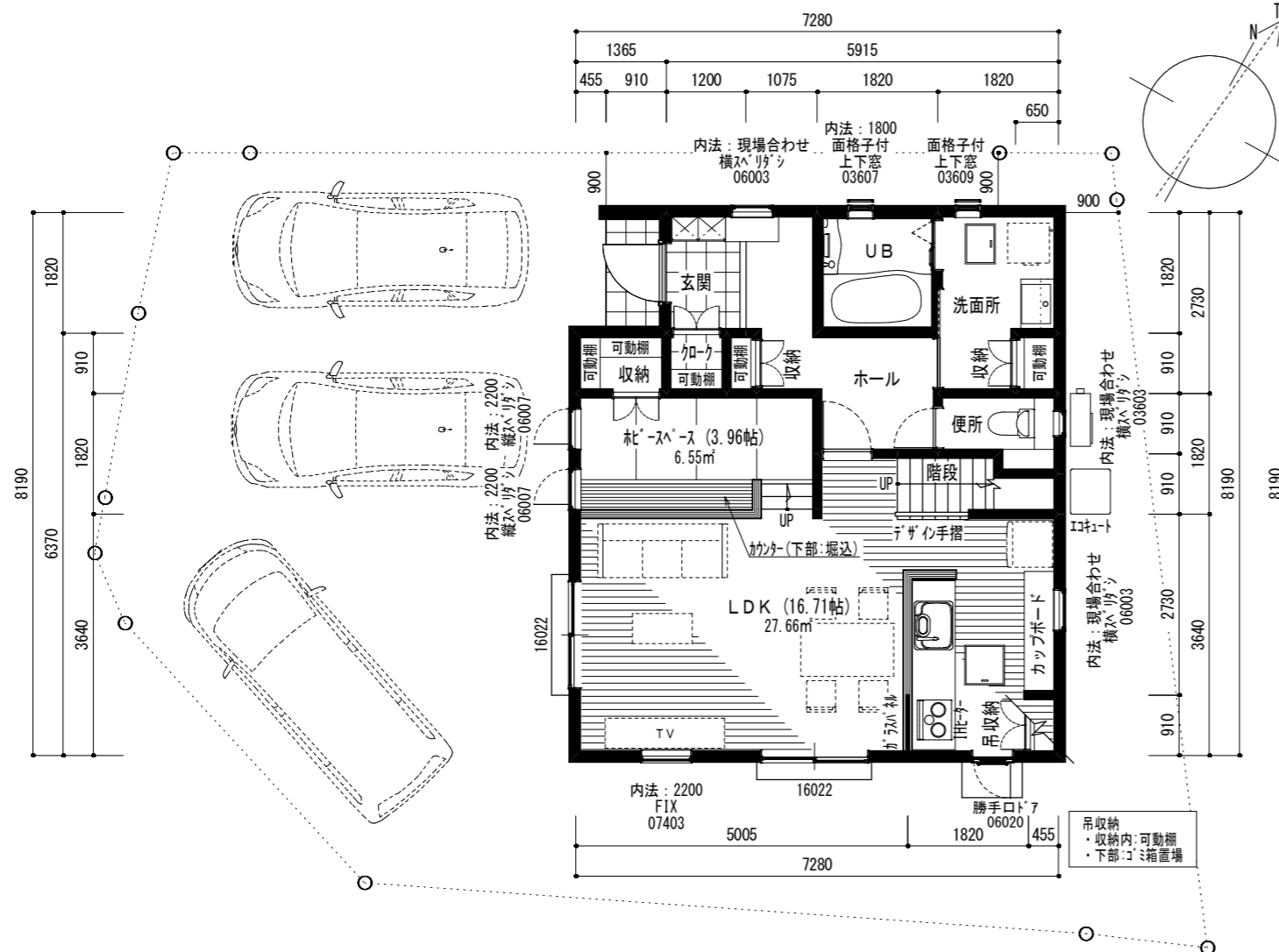
1階平面図 (プレゼン) 1/100
