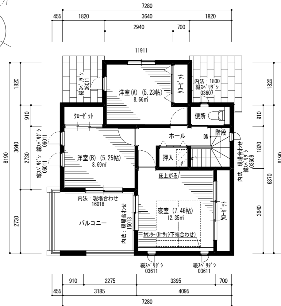
2階平面図 (プレゼン) 1/100
