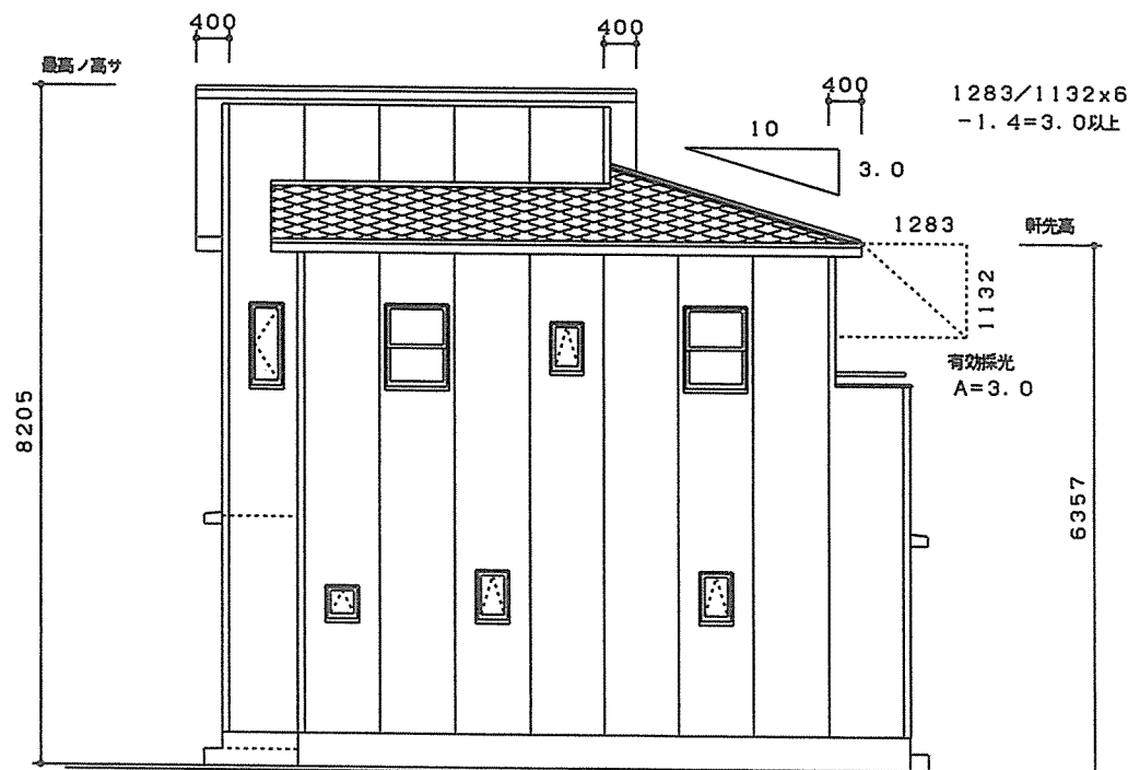
西立面図
