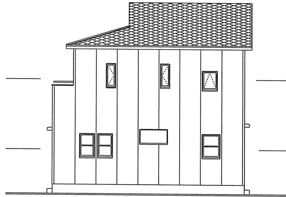
東立面図
