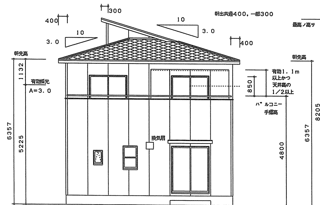
南立面図
