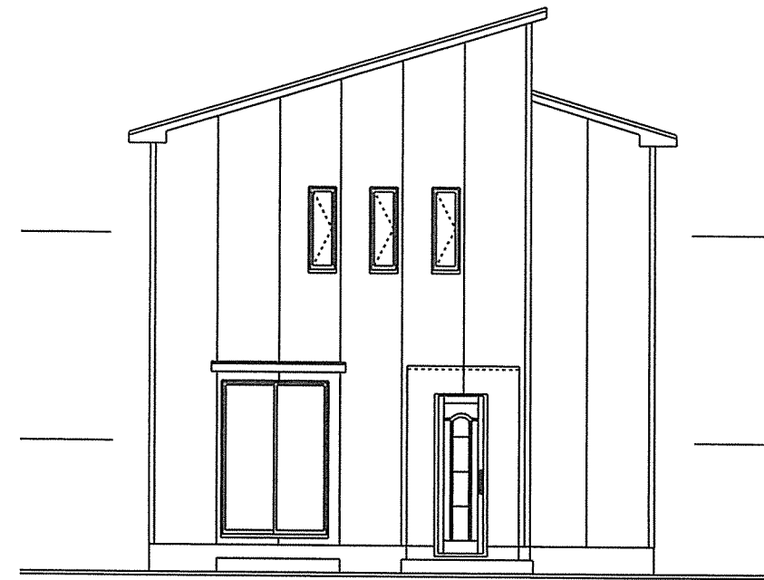
北立面図
