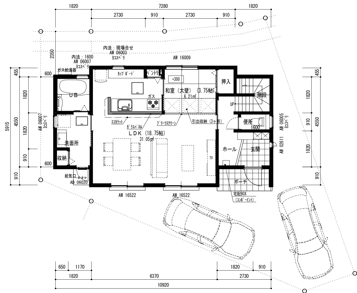
1階平面図（プレゼン） 1/100
