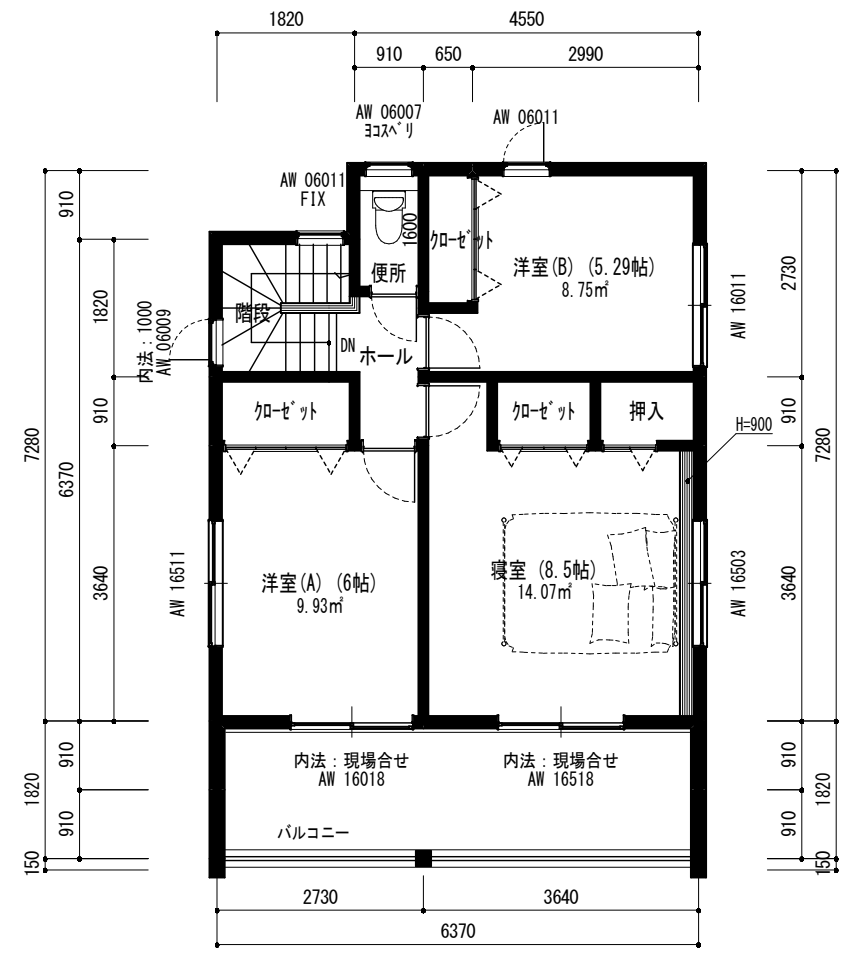
2階平面図 (プレゼン) 1/100
