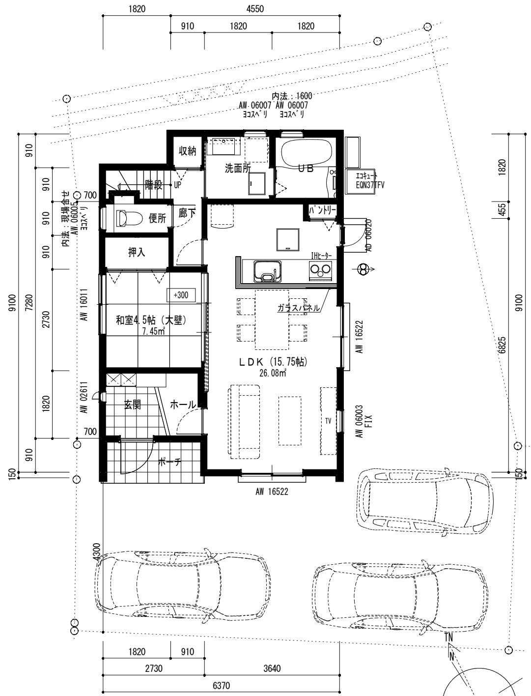
1階平面図 (プレゼン) 1/100
