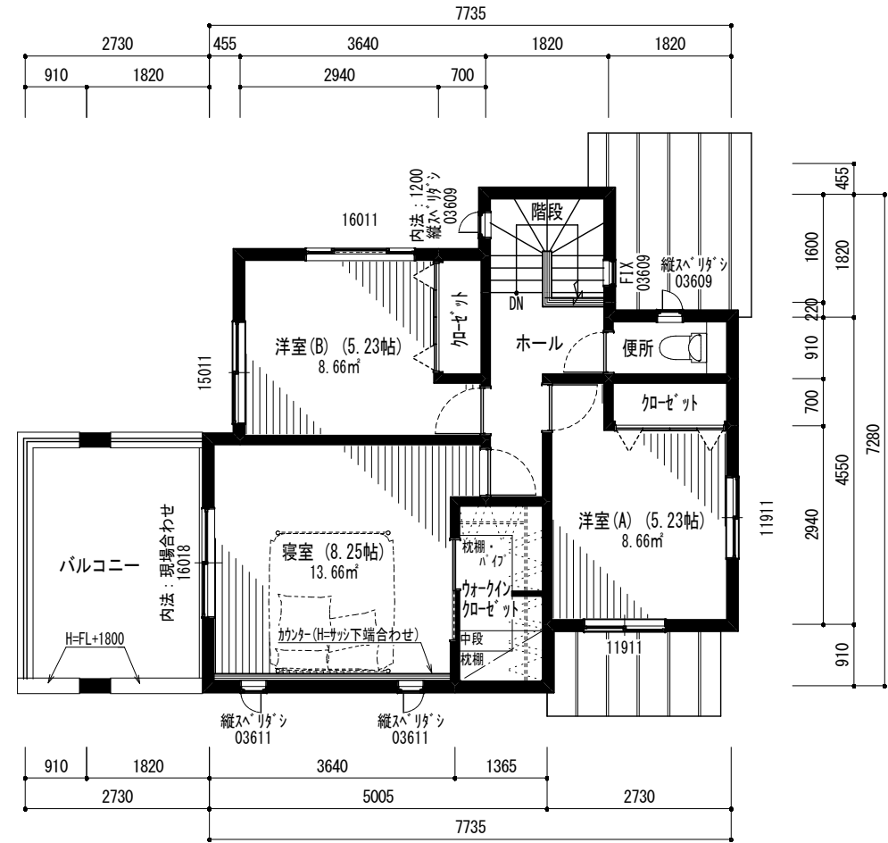
2階平面図 (フ レ ン) 1/100
