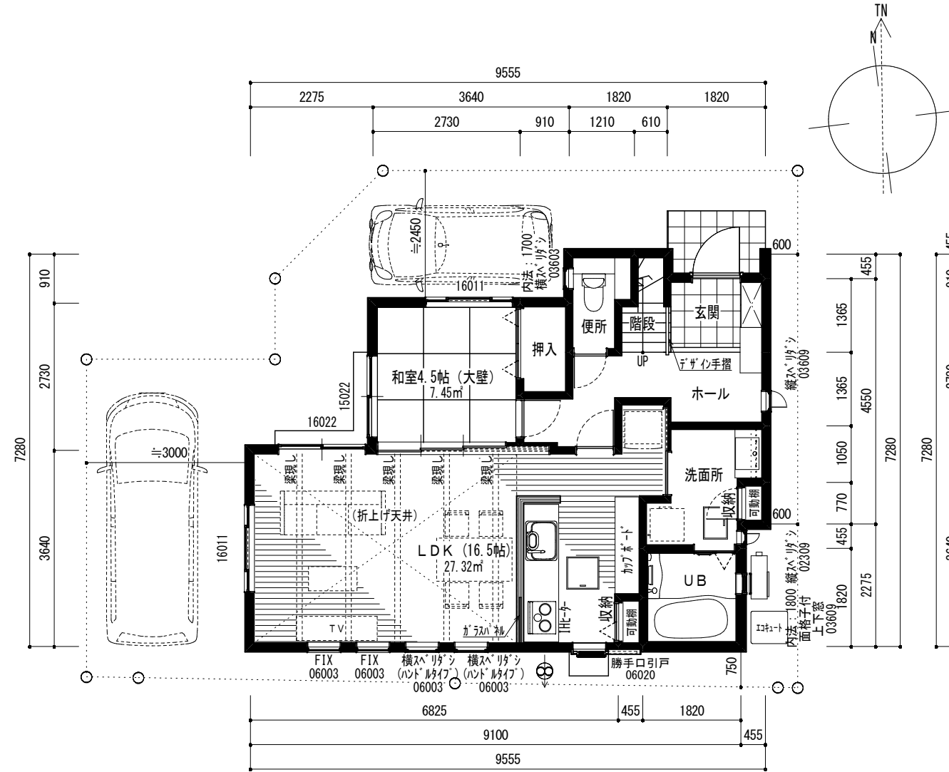
1階平面図 (フ レ ン) 1/100
