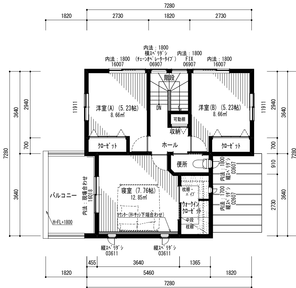
2階平面図 (プレゼン) 1/100
