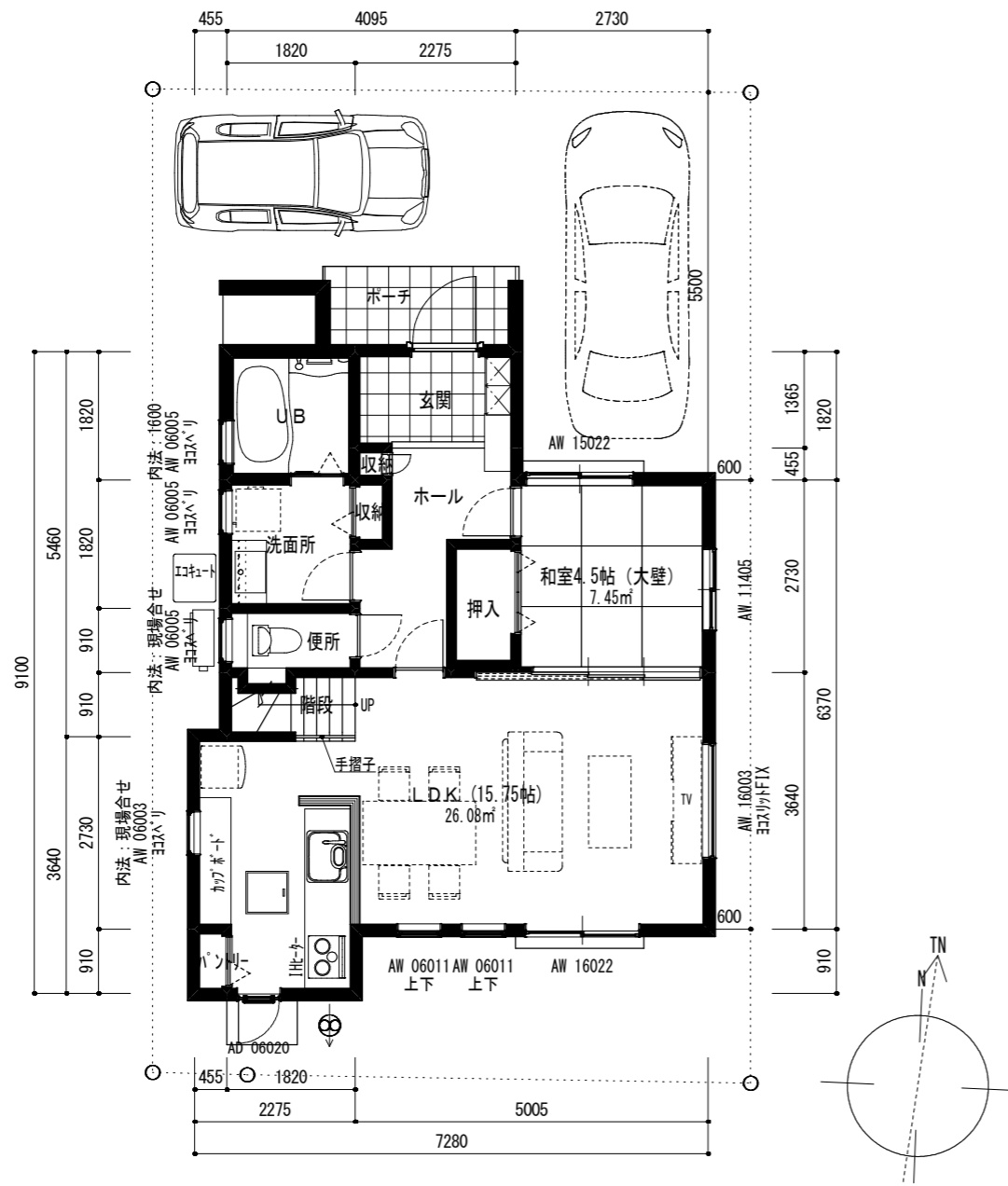
1階平面図 (プレゼン) 1/100
