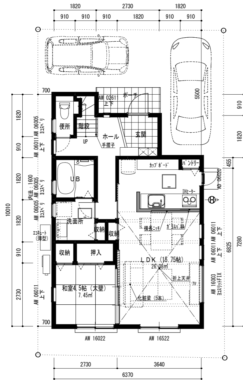
1階平面図 (プレゼン) 1/100
