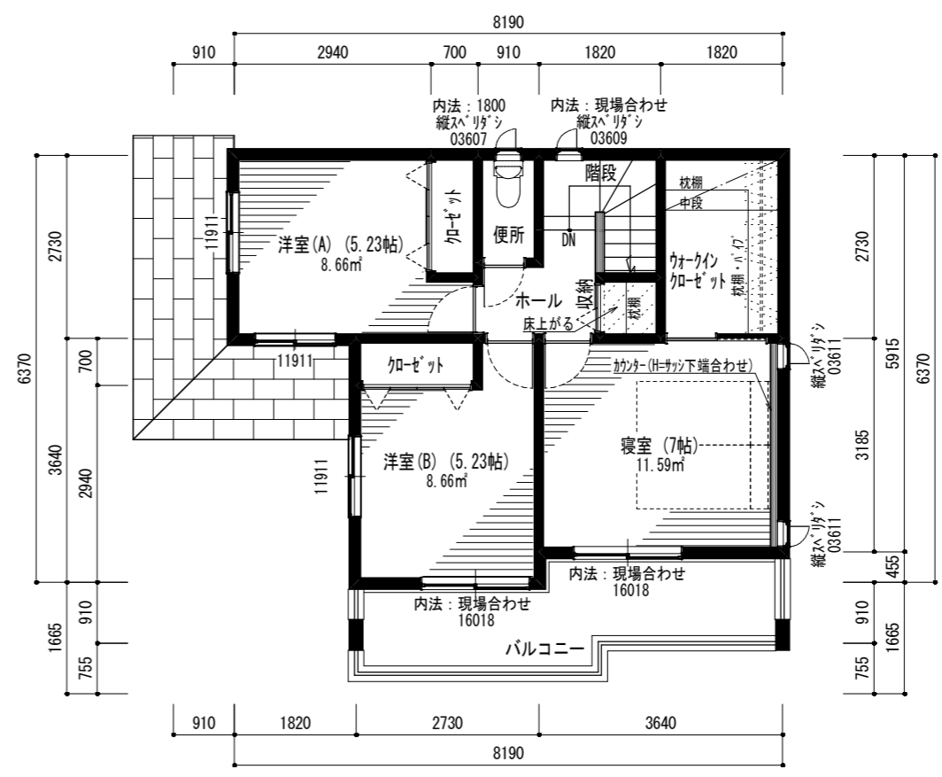
2階平面図 (プレゼン) 1/100
