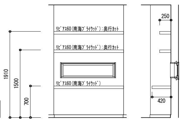
ダイニングカウンター イメージ図 1/50
