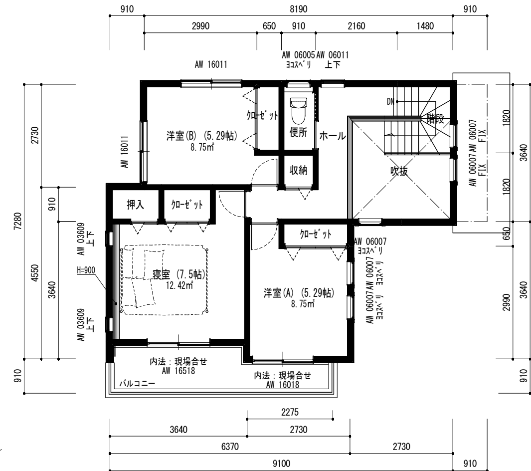
2階平面図 (プレゼン) 1/100
