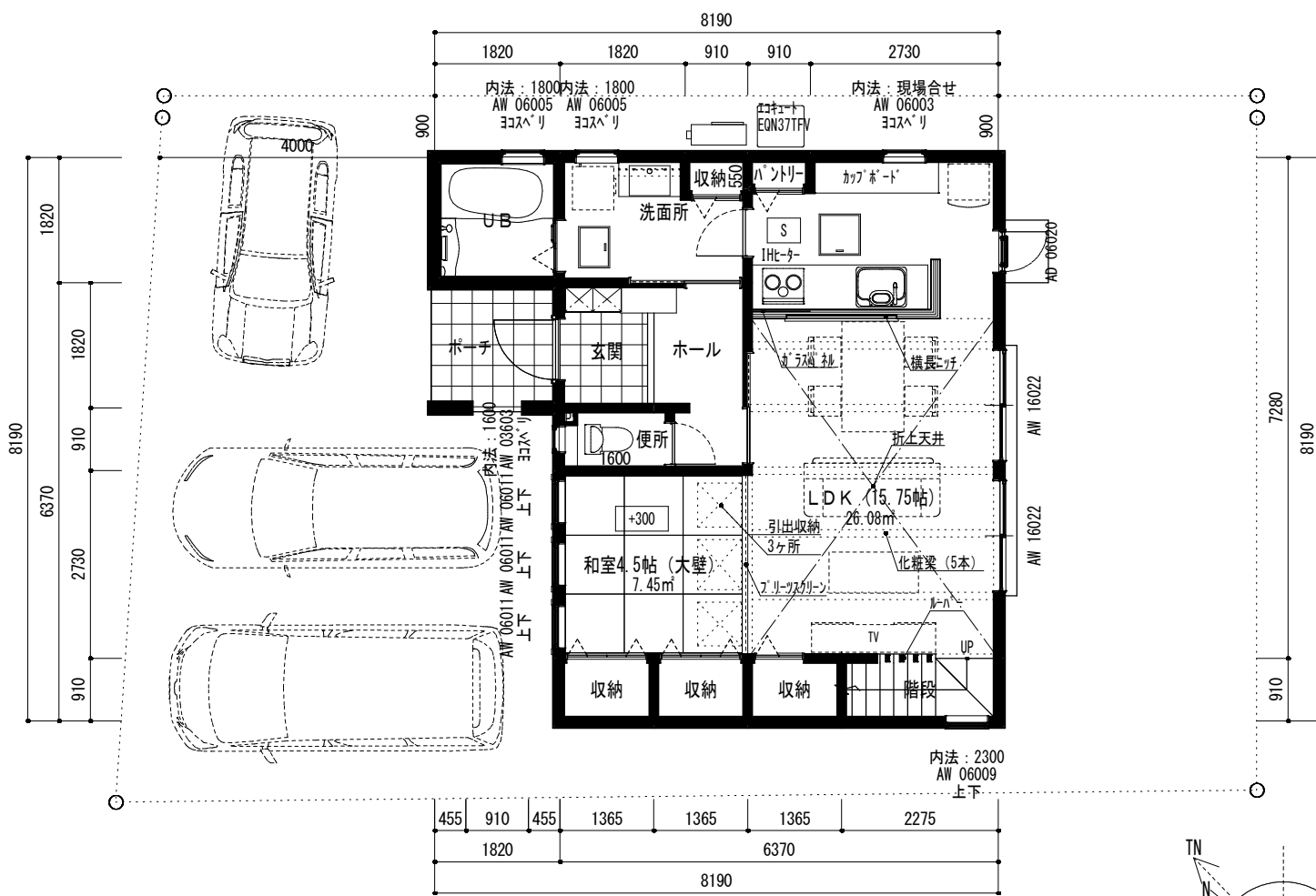
1階平面図 (プレゼン) 1/100
