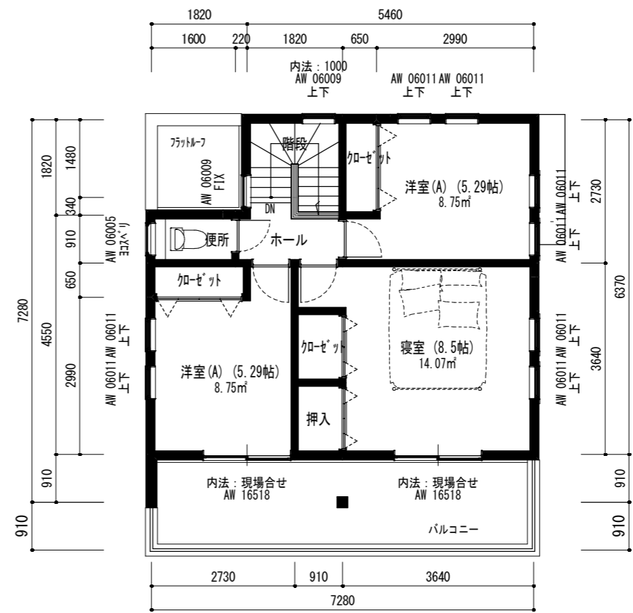
2階平面図 (プレゼン) 1/100
