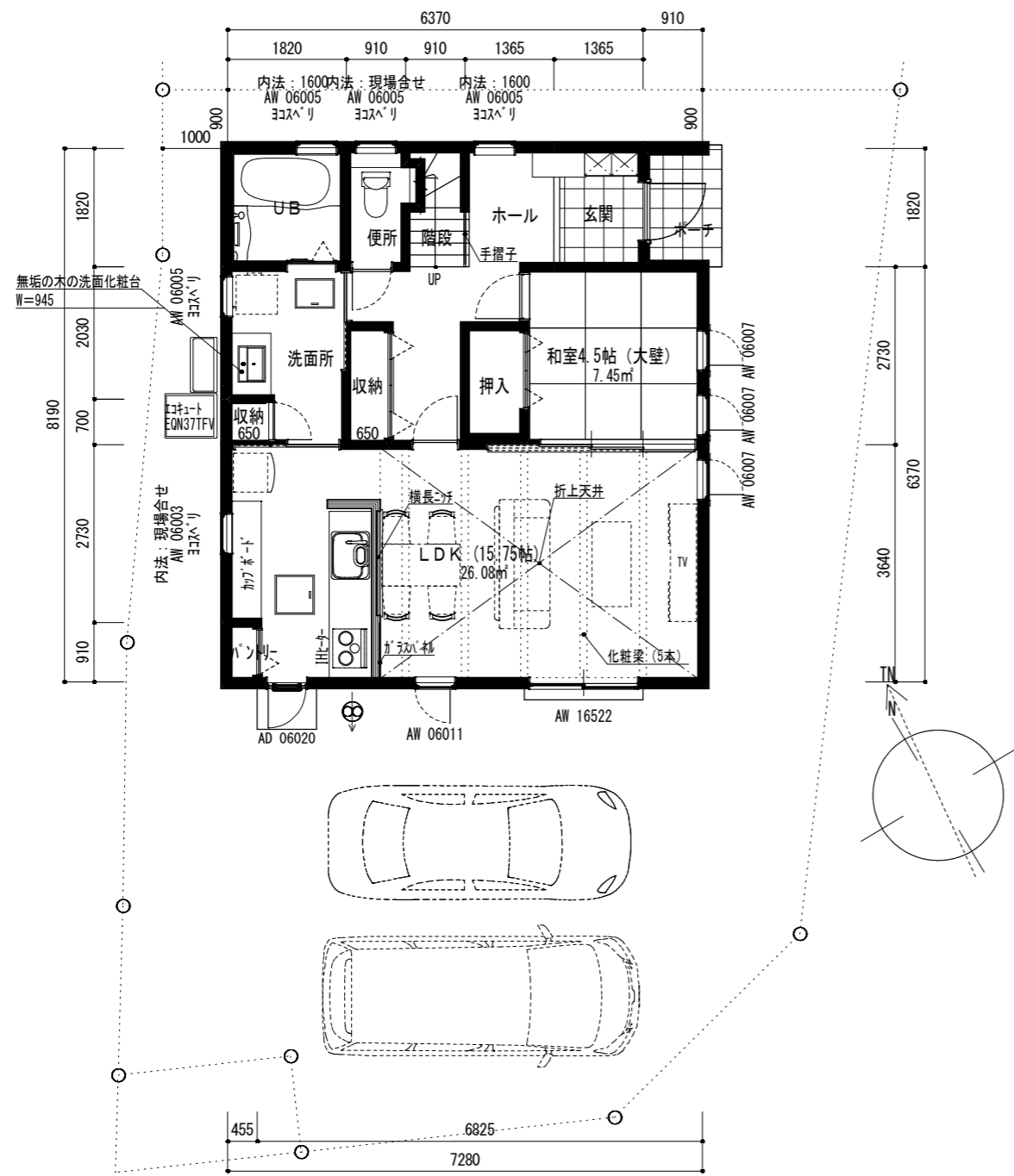
1階平面図 (プレゼン) 1/100
