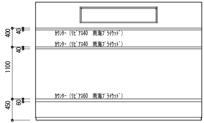
TVカウンターイメージ図 1/50
