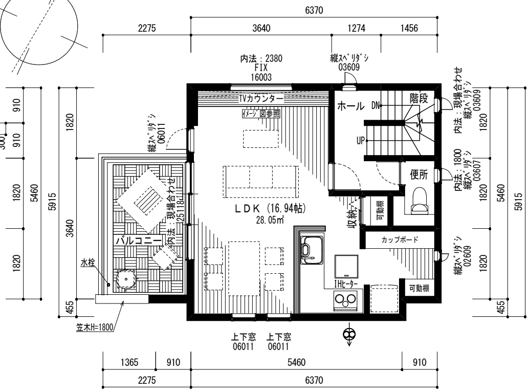
2階平面図（プレゼン） 1/100
