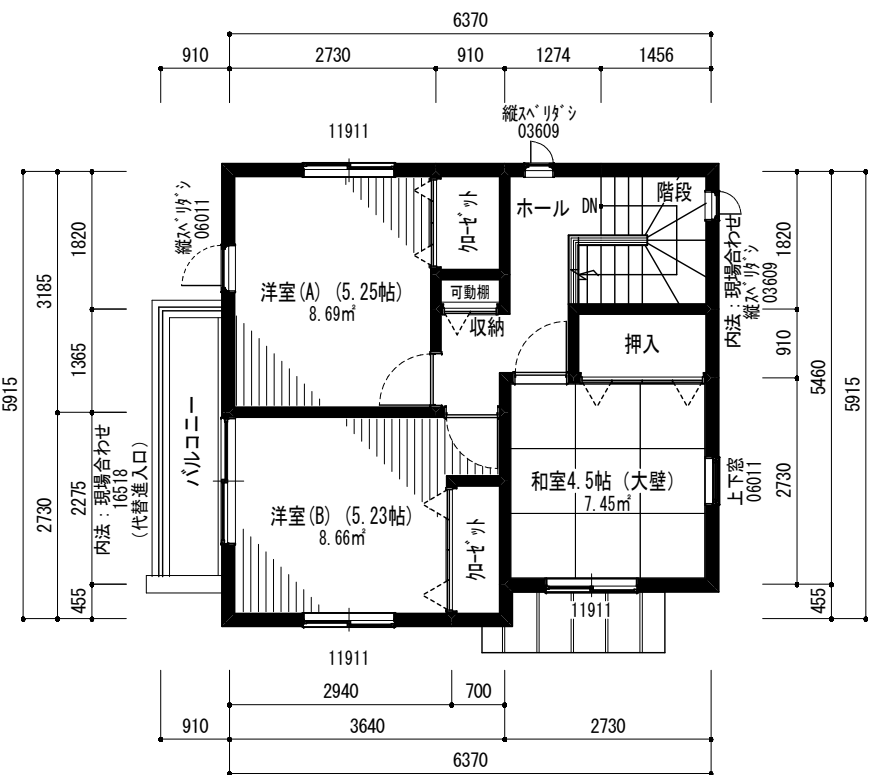
3階平面図（プレゼン） 1/100
