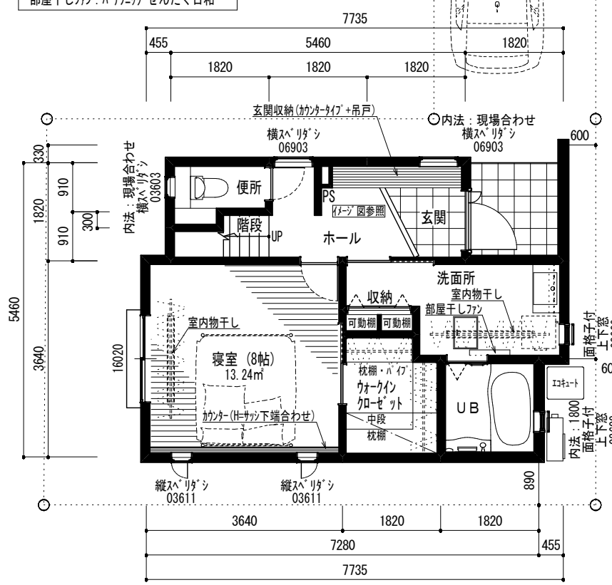
1階平面図 (プレゼン) 1/100
