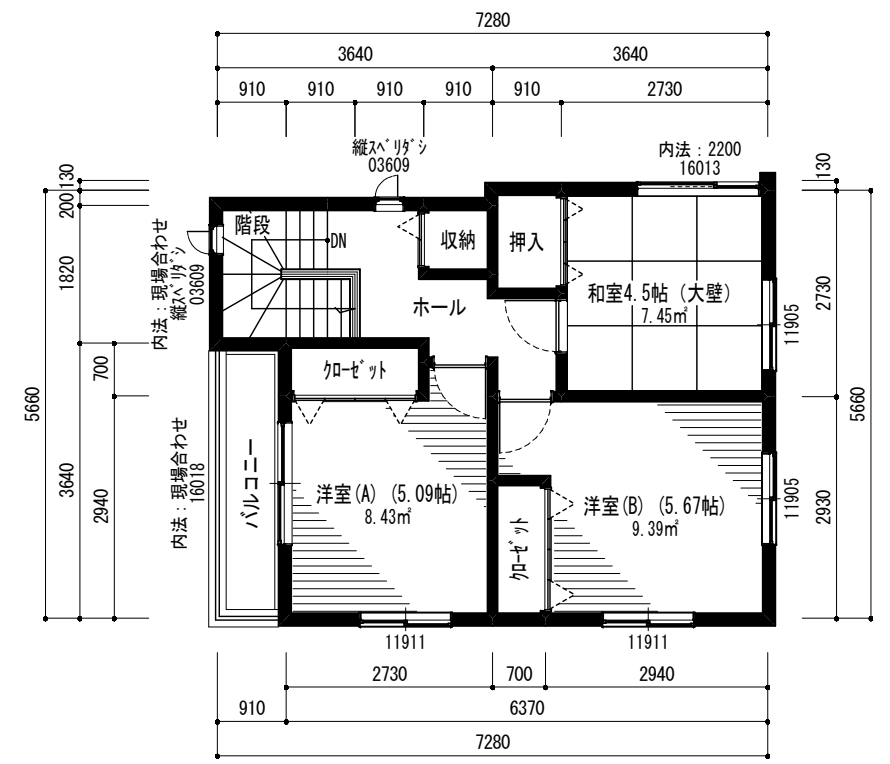
3階平面図 (プレゼン) 1/100
