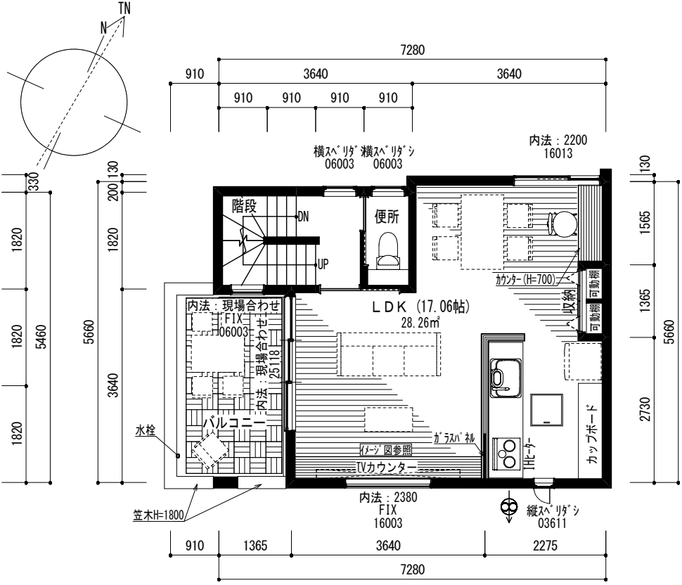
2階平面図 (プレゼン) 1/100
