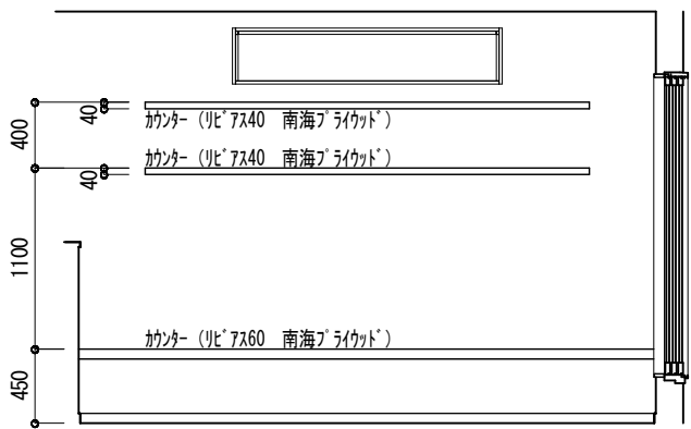
TVカウンター イメージ展開図 1/50
