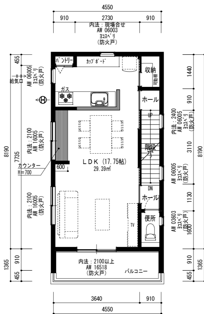
2階平面図 (プレゼン) 1/100
