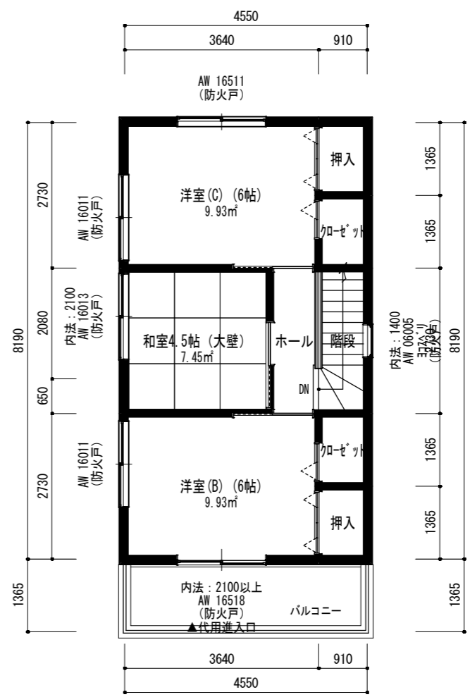
3階平面図 (プレゼン) 1/100
