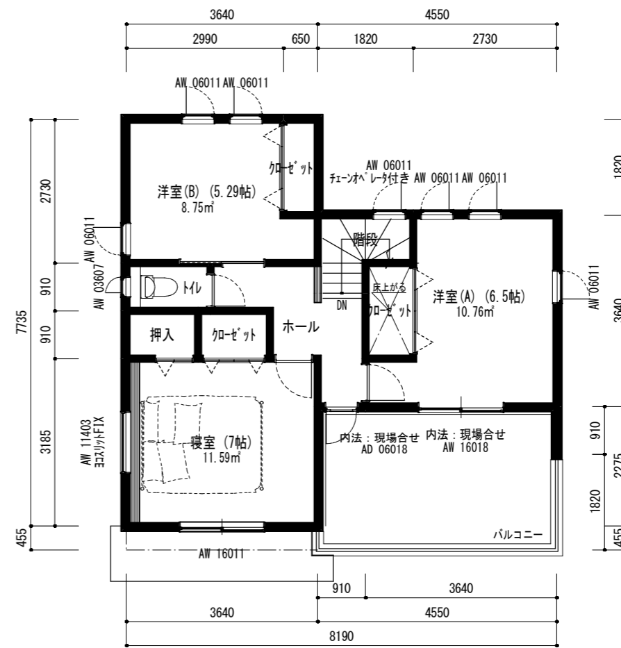
2階平面図 (プレゼン) 1/100
