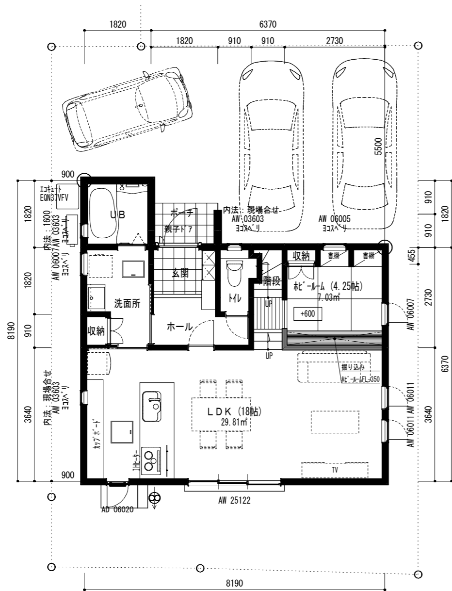
1階平面図 (プレゼン) 1/100
