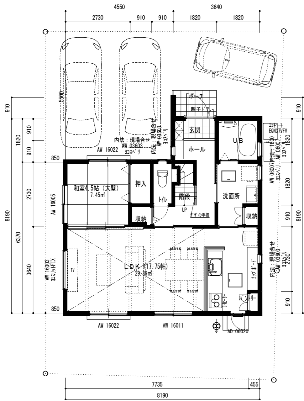
1階平面図 (プレゼン) 1/100
