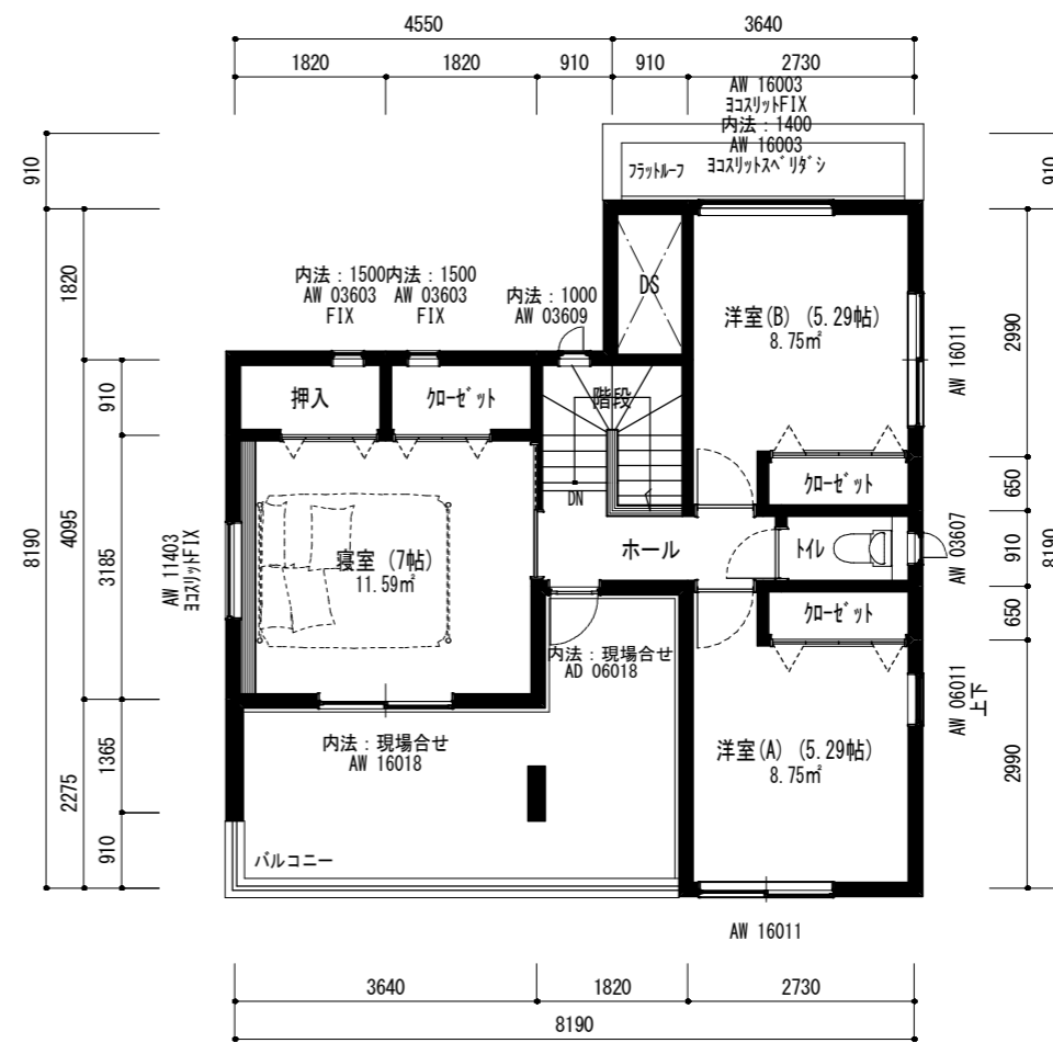
2階平面図 (プレゼン) 1/100
