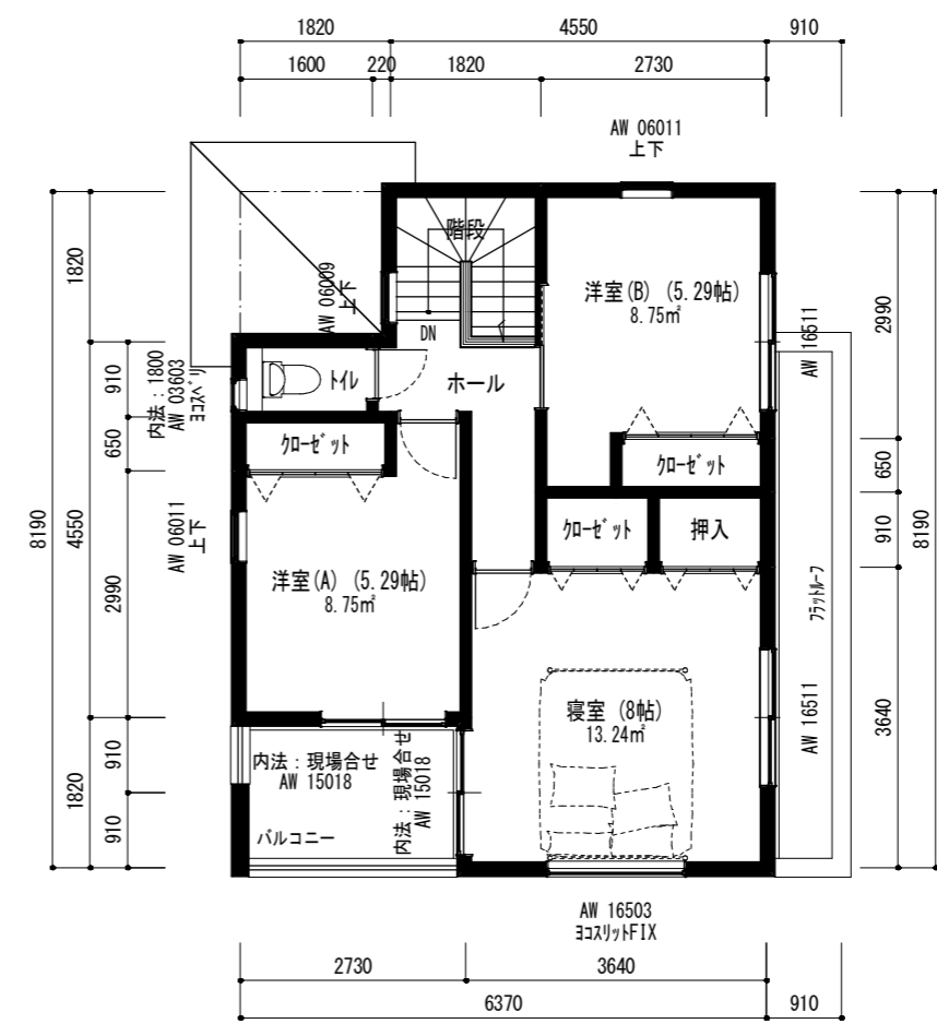
2階平面図 (プレゼン) 1/100
